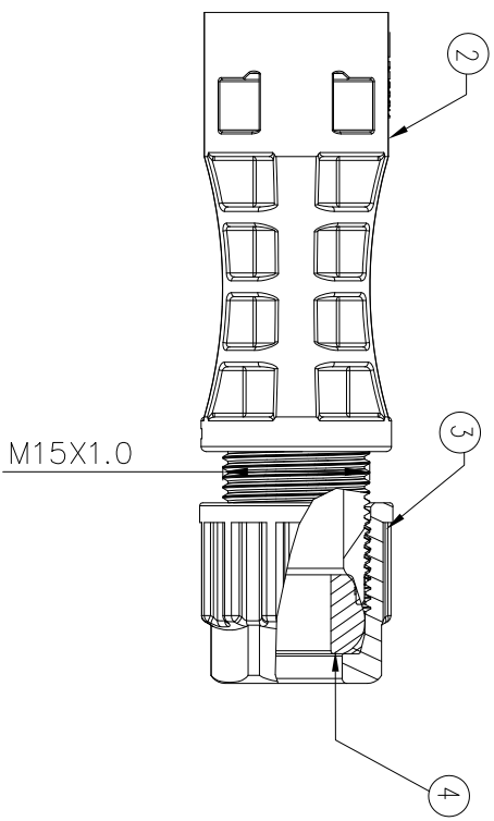
截面 B-B
